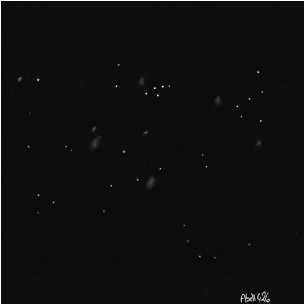
Abell426 - PERSEE / Groupe de galaxies Dobson : 403mm Grossissement : 224x Filtre : Aucun Date : 14/01/2018 21:10 Lieu : Vieux Berquin(Nord) Ciel moyen
