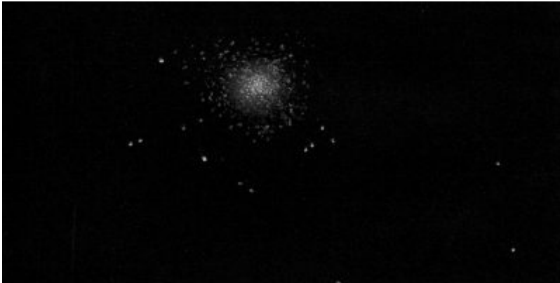
M62-SERPENTAIRE / Dobson : 403mm Grossissement : 225x Filtre : Aucun Lieu : Pontenx les forges (Landes) Date : 10/08/2015 23:15 Ciel très bon
