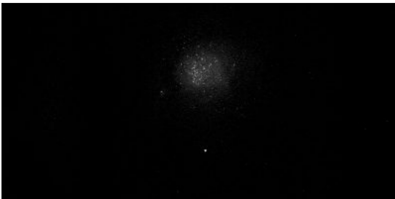
M79-LIEVRE / M79 Amas globulaire Constellation : Lièvre Dobson : 403mm Grossissement : 280x Filtre : Aucun Lieu : Landas (Nord) Date : 16/02/2016 20:20 Ciel très moyen 15° au dessus de l'horizon
