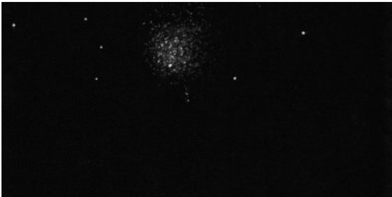
M107-SERPENTAIRE / Dobson : 403mm Grossissement : 225x Filtre : Aucun Lieu : Pontenx les forges (Landes) Date : 09/08/2015 23:00 Ciel très bon
