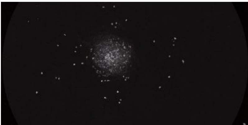
M15-PEGASE / Dobson : 403mm Grossissement : 225x Filtre : aucun Lieu : Gruson (Nord) Date : 04/09/2014 00:30 Ciel moyen
