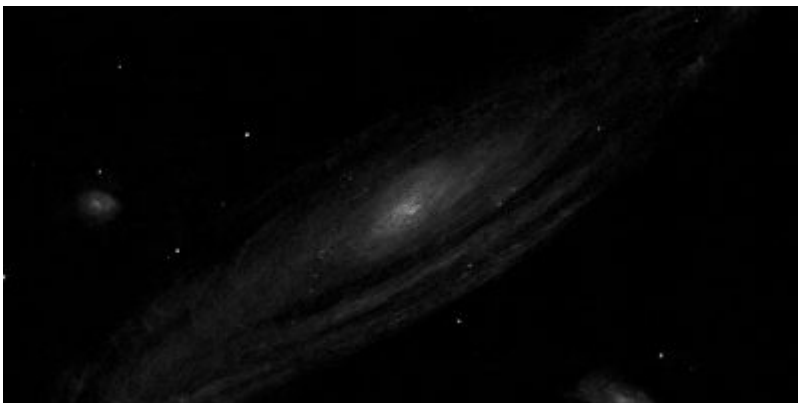
M31-PEGASE / Dobson : 403mm Grossissement : 85x Filtre : Aucun Lieu : Pontenx les forges (Landes) Date : 21/08/2015 3:00 Ciel parfait
