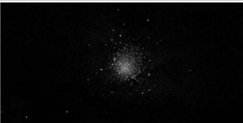
M2-VERSEAU / Dobson : 403mm Grossissement : 225x Filtre : OIII Lieu : Landas (Nord de la France) Date : 04/03/2013 21:00 Ciel moyen
