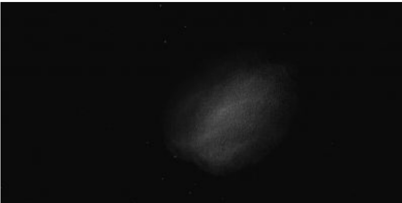
M1-TAUREAU / Dobson : 403mm Grossissement : 225x Filtre : OIII Lieu : Landas (Nord de la France) Date : 04/03/2013 21:00 Ciel moyen
