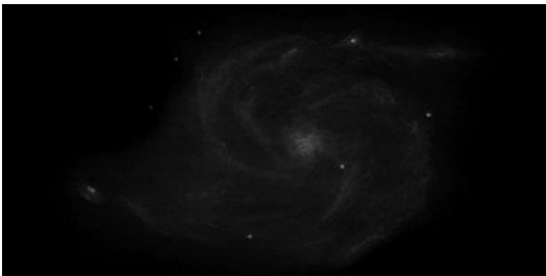
M101-GRANDE OURSE / Dobson : 403mm Grossissement : 225x Filtre : Aucun Lieu : Froidestrées (Aines) Date : 25/03/2012 02:40 Ciel très bon
