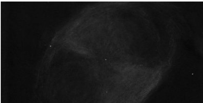
M27-PETIT RENARD / Dobson : 403mm Grossissement : 225x Filtre : OIII Lieu : Pontenx les forges (Landes) Date : 19/08/2015 1:00 Ciel parfait
