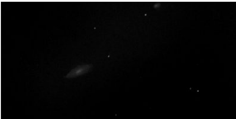
M59-IC809-VIERGE / Galaxies Dobson : 403mm Grossissement : 225x Filtre : CLS Lieu : Landas(Nord 59) Date : 30/04/2017 0:40 Ciel moyen
