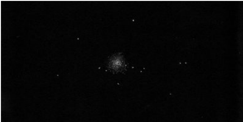
M19-SERPENTAIRE / Dobson : 403mm Grossissement : 225x Filtre : Aucun Lieu : Pontenx les forges (Landes) Date : 10/08/2015 23:30 Ciel bon
