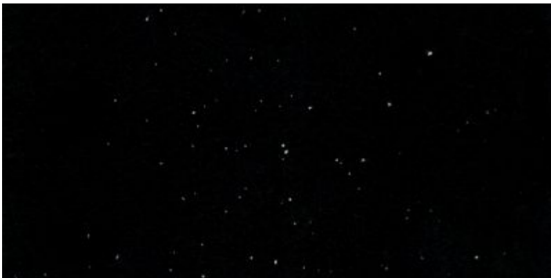
M36-COCHER / AMAS ouvert M36 Constellation : Cochér Dobson : 403mm Grossissement : 140x Filtre : Aucun Lieu : Landas (Nord) Date : 03/12/2016 23:30 Ciel moyen
