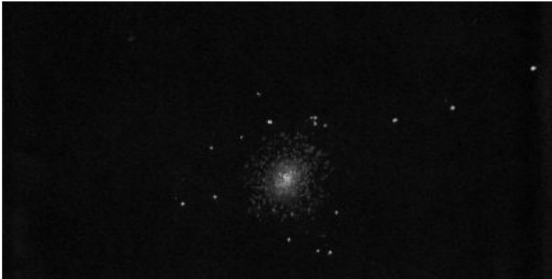
M80-SAGITTAIRE / Dobson : 403mm Grossissement : 225x Filtre : Aucun Lieu : Pontenx les forges (Landes) Date : 10/08/2015 22:45 Ciel très bon
