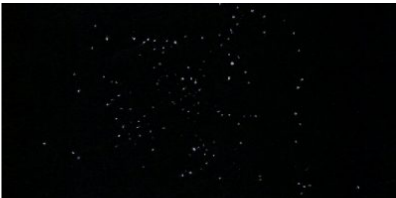
M11-ECU SOBIESKI / Dobson : 403mm Grossissement : 140x Filtre : Aucun Lieu : Landas(Nord) Date : 11/10/2015 20:40 Ciel bon
