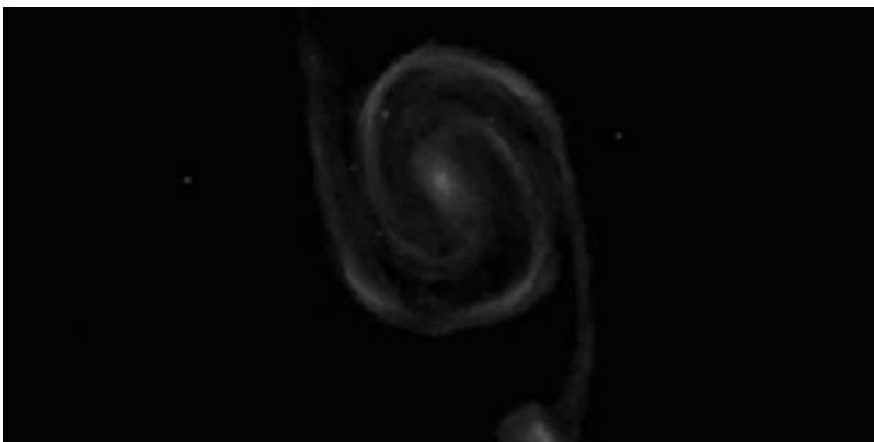
M51-CHIENS DE CHASSE / Dobson : 403mm Grossissement : 225x Filtre : Aucun Lieu : Froidestrées (Aines) Date : 16/05/2012 02:50 Ciel très bon
