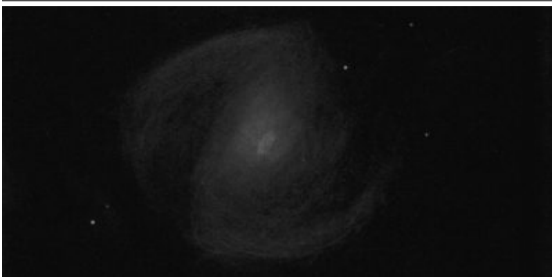
M74-POISSONS / Dobson : 403mm Grossissement : 225x Filtre : CLS Lieu : Pontenx les forges (Landes) Date : 19/08/2015 3:30 Ciel très bon
