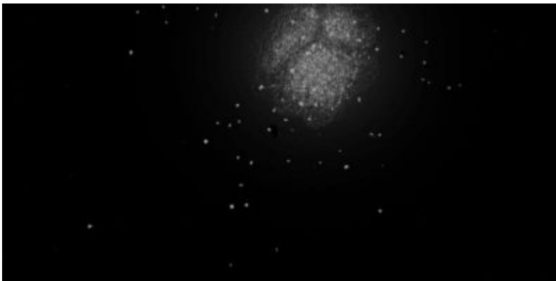
M13-HERCULE / Dobson : 403mm Grossissement : 450x Filtre : aucun Lieu : Landas (Nord) Date : 21/04/2013 01:30 Ciel moyen
