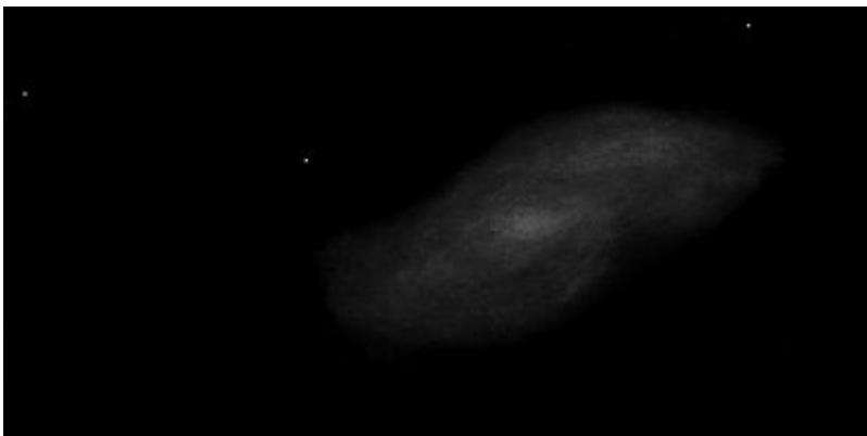
M66-LION / Dobson : 403mm Grossissement : 225x Filtre : Aucun Lieu : Landas (Nord) Date : 14/04/2012 23:45 Ciel bon
