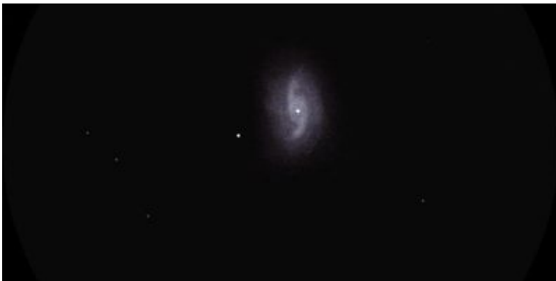
M77-BALEINE / Dobson : 403mm Grossissement : 280x Filtre : Aucun Lieu : Landas (NORD) Date : 30/11/2013 22:20 Ciel moyen
