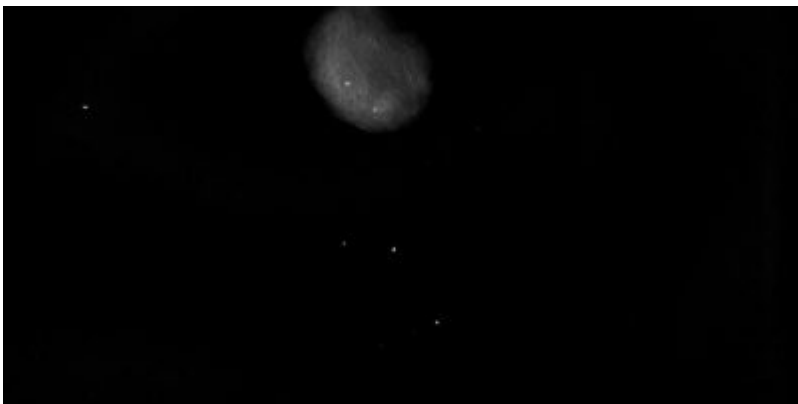
M78-ORION / Dobson : 403mm Grossissement : 140x Filtre : UHC Lieu : Gruson (Nord) Date : 02/02/2013 22:00 Ciel très moyen
