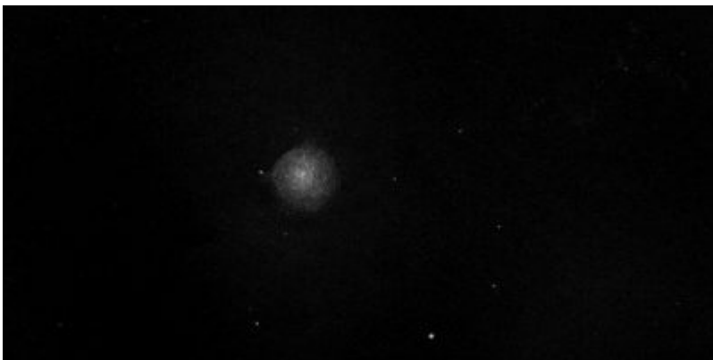
M54-SAGITTAIRE / Amas Globulaire Dobson : 403mm Grossissement : 225x Filtre : Aucun Lieu : Pontenx les Forges(LANDES-40) Date : 25/08/2017 22:10 Ciel très bon Mais beaucoup de turbulence
