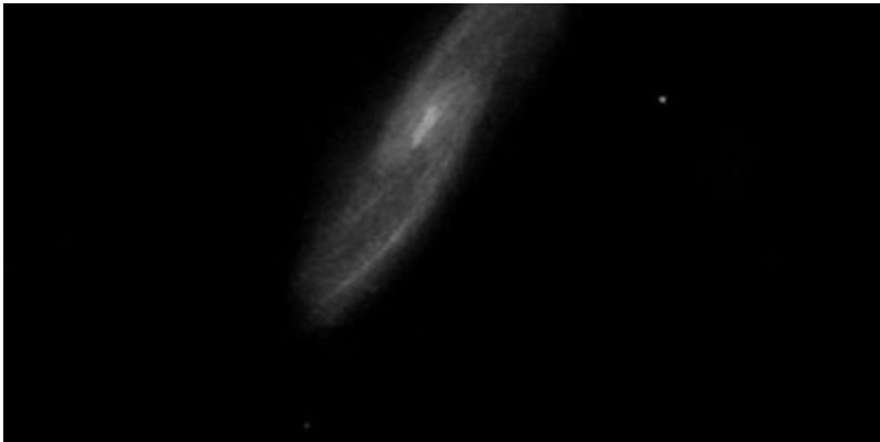
M106-CHIENS DE CHASSE / Dobson : 403mm Grossissement : 225x Filtre : Aucun Lieu : Landas (Nord) Date : 25/01/2014 22:50 Ciel très moyen
